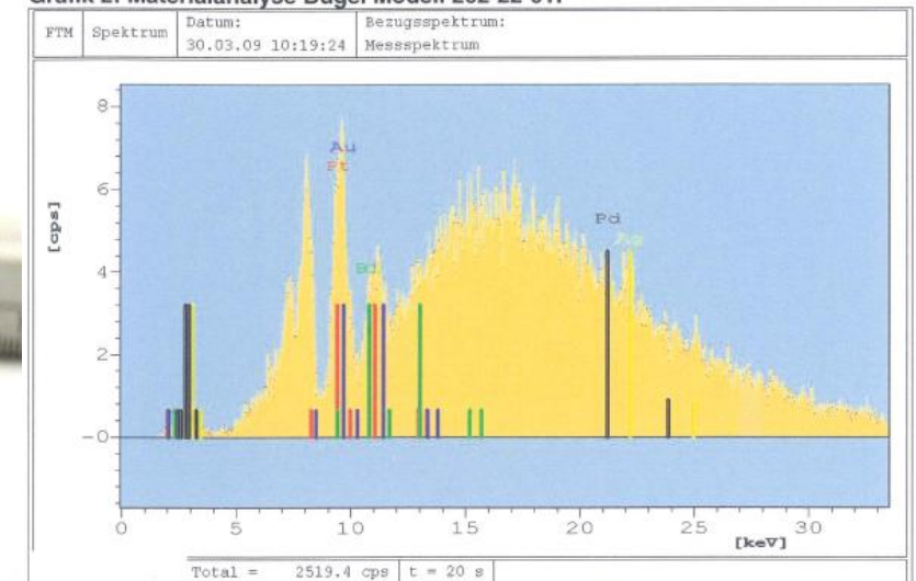
Grafik 2: Materialanalyse Bügel Modell 202-22-01P
